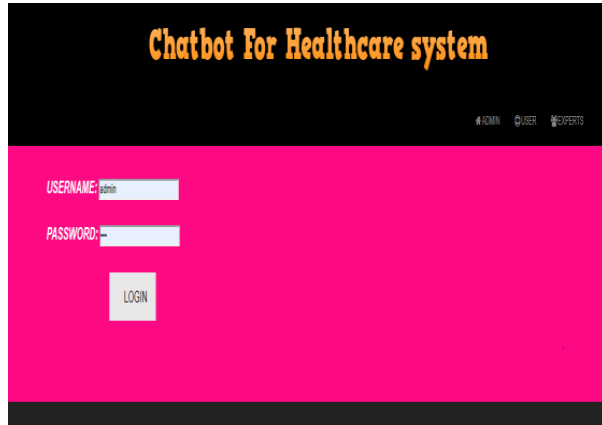
Fig. 2: Login page
